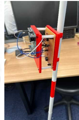
電子白杖(開発中) (つくば工科高校)
